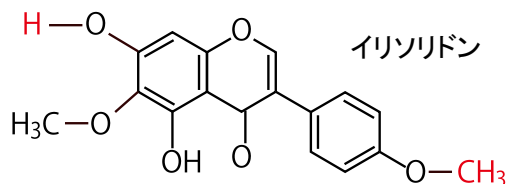
図1 葛花イソフラボンの構造
